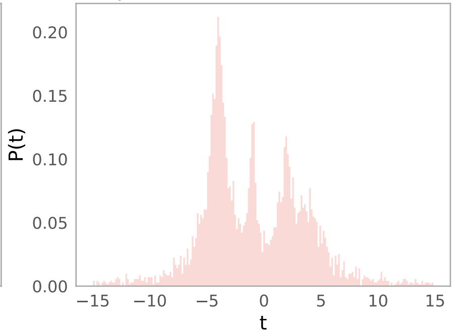
plt.hist(t, bins=200)
