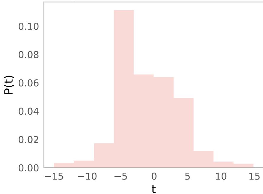
plt.hist(t, bins=10)
